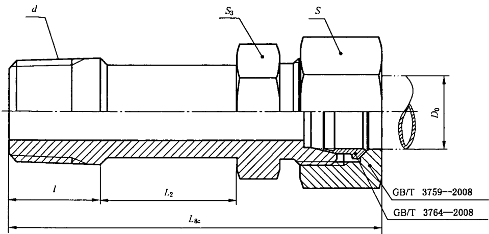
图 1 卡套式锥螺纹直通长管接头
